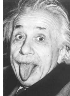
Albert Einstein
